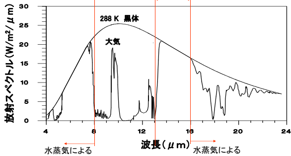
黒体と大気から射出される熱放射スペクトル
